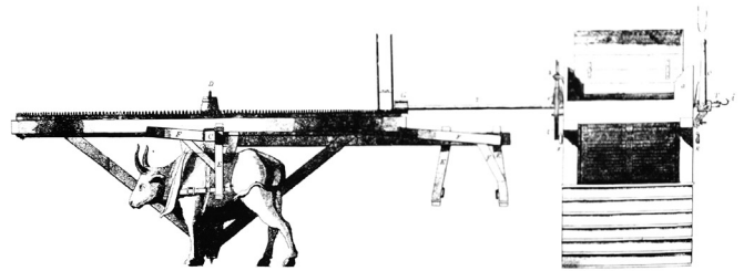
Bild 10. Tröskverk med vandring. Överst principskiss med dragdjur som vandrar runt och driver vertikalaxeln. En vinkelväxel överför kraften till en horisontell axel som driver tröskverket.
